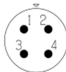
図.プラグのピン番号
